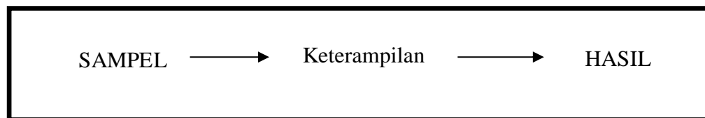
Gambar. 1. Desain Penelitian
